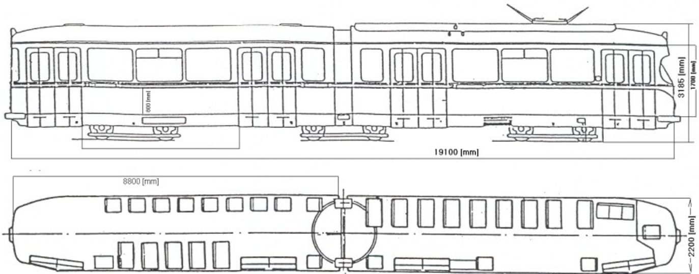
Fig.8 - Tramvai GT6
