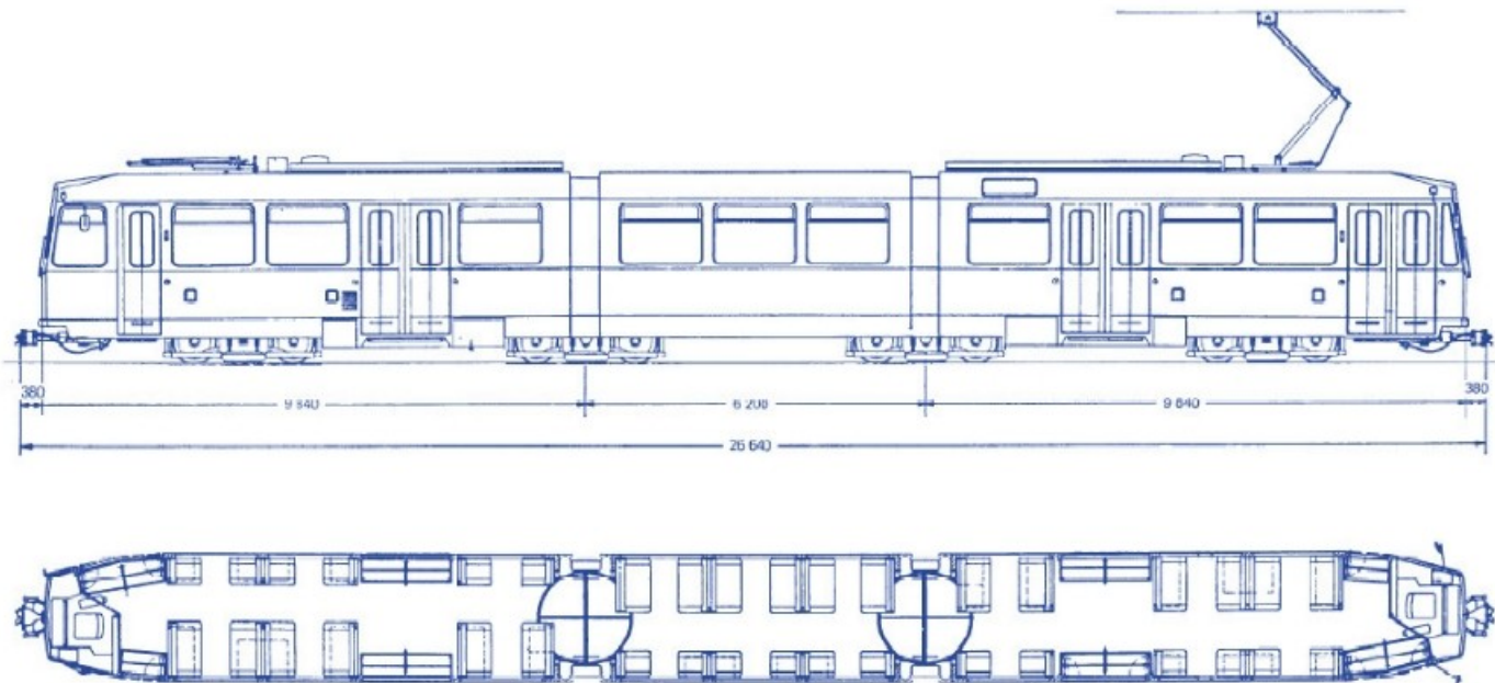
Fig.10 - Tramvai GT8
