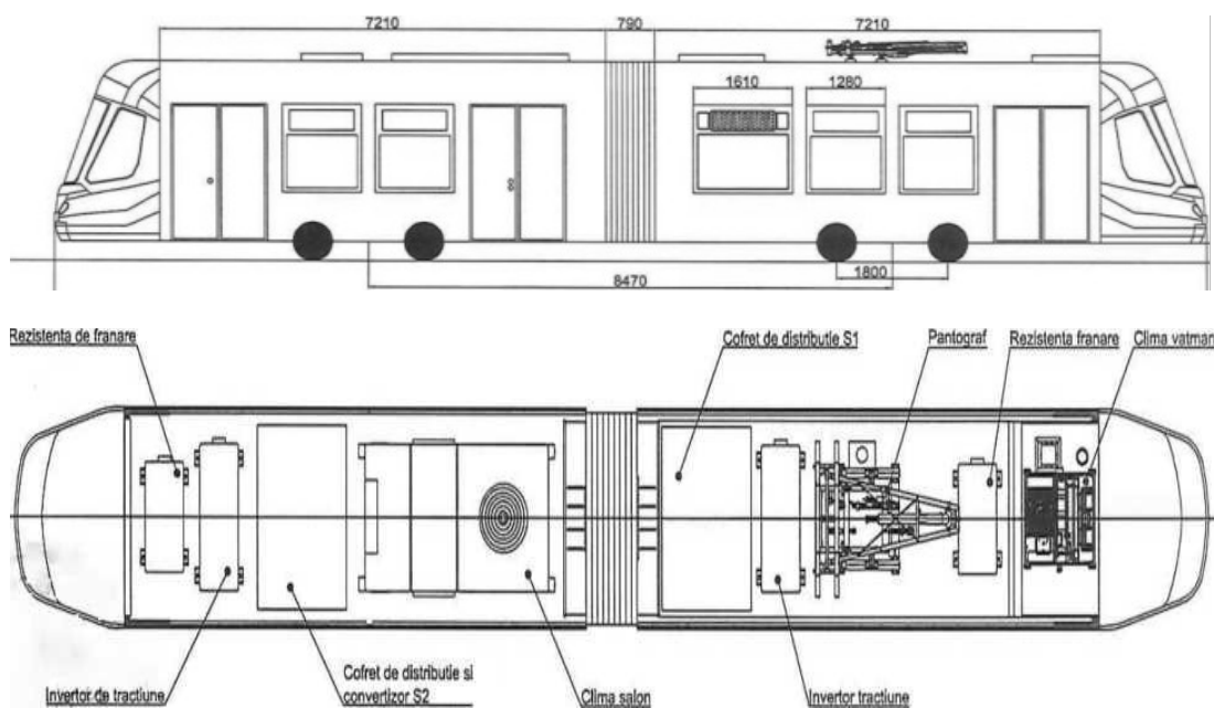
Fig.12 - Tramvai Imperio
