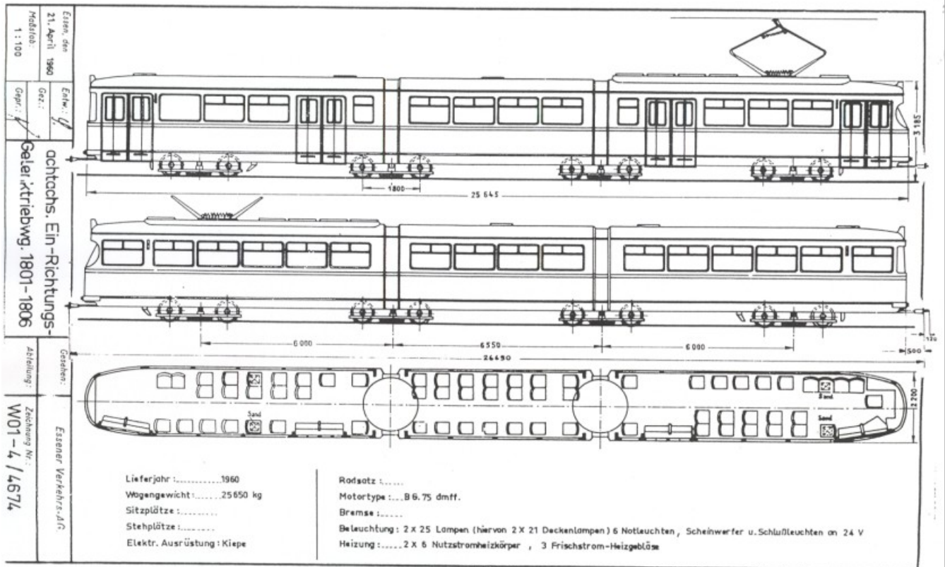
Fig.10 - Tramvai GT8
